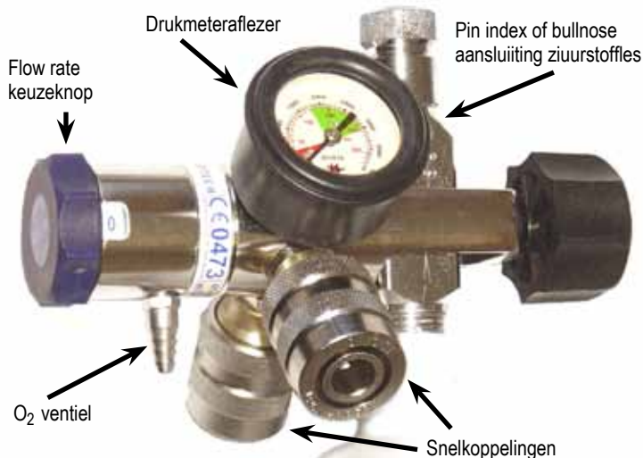
Model: bull nose met 2 snelkoppelingen 677-0001-20
